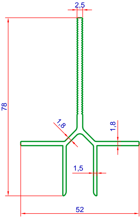
8604 0.743 kg/m
