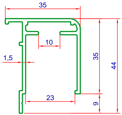
8602 0.530 kg/m
