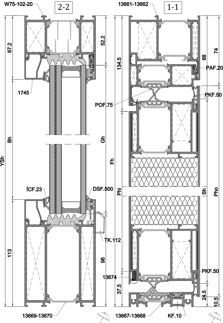
Tek Kanat-Yan Sabit Dışa Açılır SINGLE SASH SIDE FIXED OPENING OUTWARD
