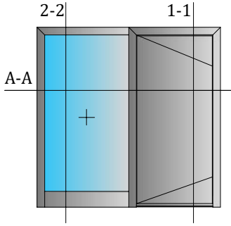
Tek Kanat-Yan Sabit Dışa Açılır SINGLE SASH SIDE FIXED OPENING OUTWARD
