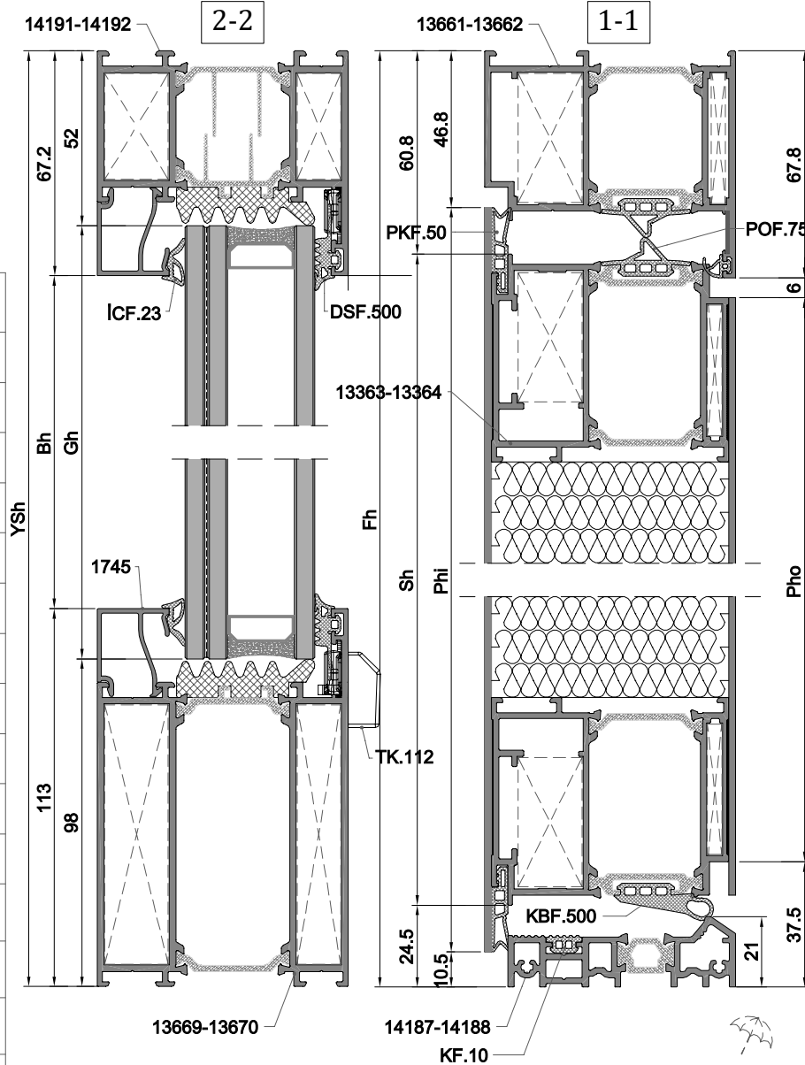
Tek Kanat-Yan Sabit İçe Açılır SINGLE SASH SIDE FIXED OPENING INWARD
