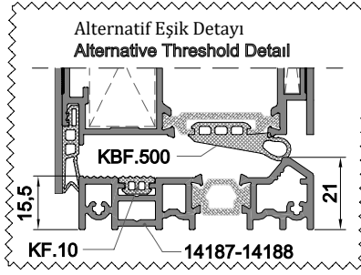
Tek Kanat - İç Açılır SINGLE SASH - OPENING INWARD
