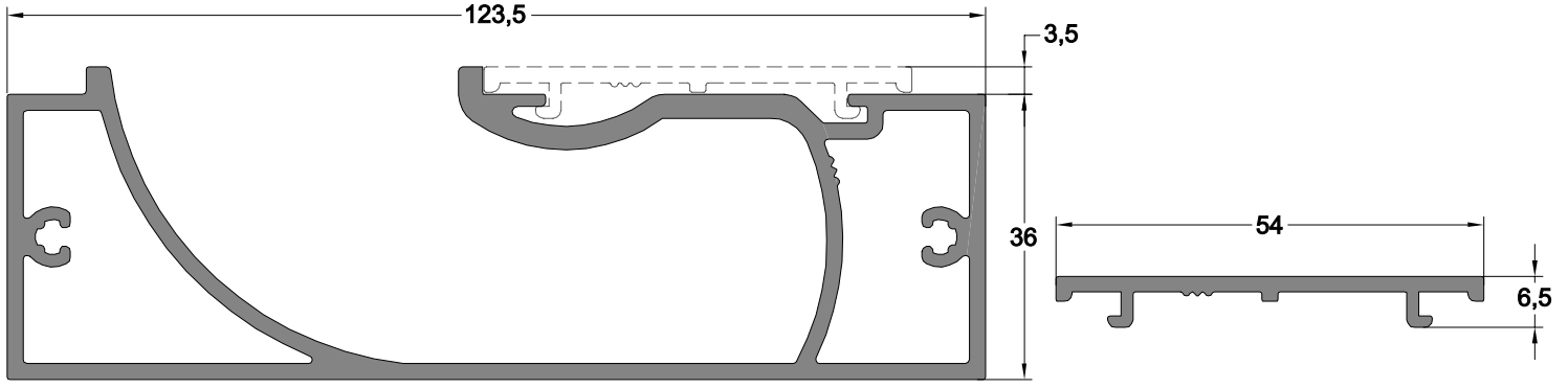
Gizli Kol Profili HIDDEN HANDLE PROFILE
