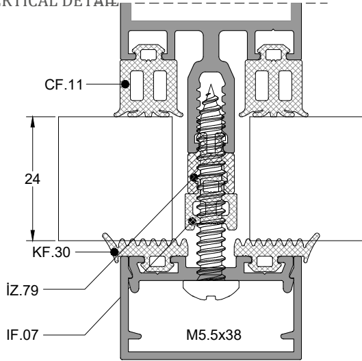
DÜŞEY DETAYI VERTICAL DETAIL
